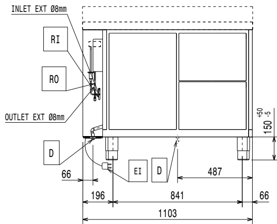
Zij aanzicht
