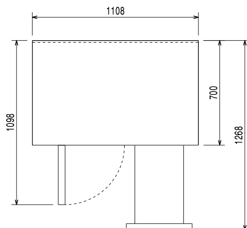
Boven aanzicht
